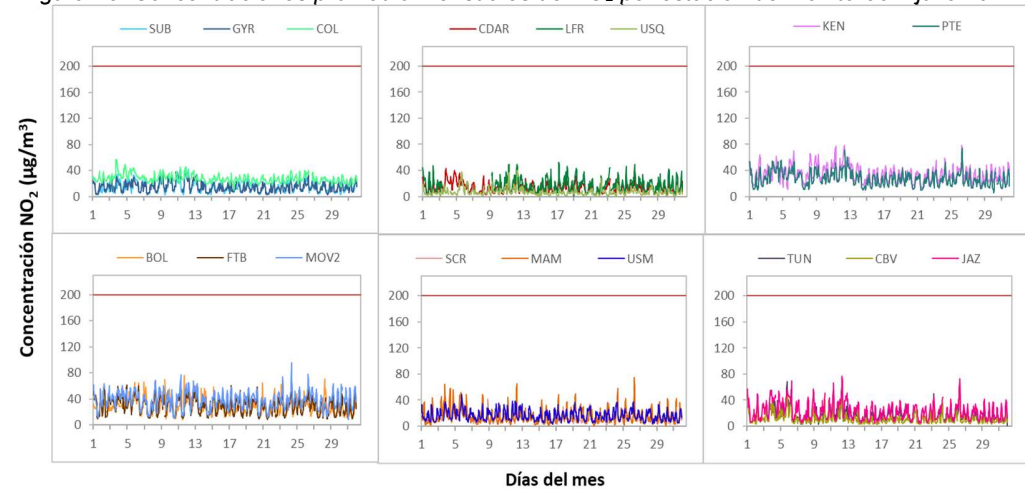
Figura 16. Concentraciones promedio mensuales de NO 2 por estación de monitoreo – julio 2024.
