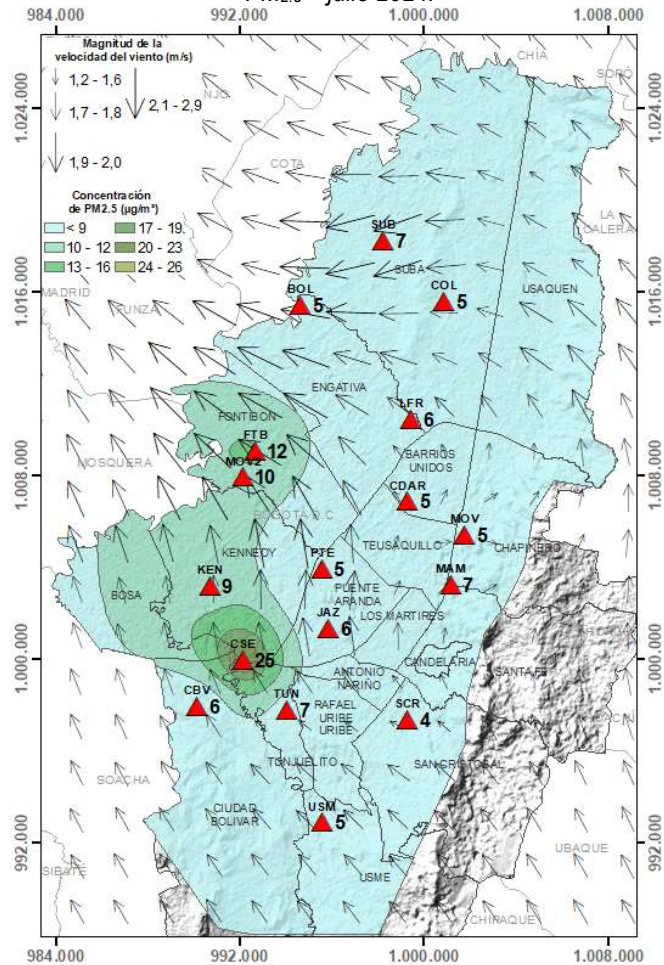
Figura 4. Distribución espacial concentraciones mensuales PM 2.5 – julio 2024.
