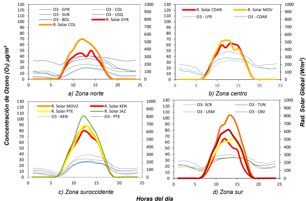
Figura 12. Comportamiento horario de las concentraciones de O 3 (µg/m 3 ) y su relación con la Radiación Solar entrante (W/m 2 ) julio 2024. a) zona norte, b) zona centro, c) zona suroccidente y d) zona sur
