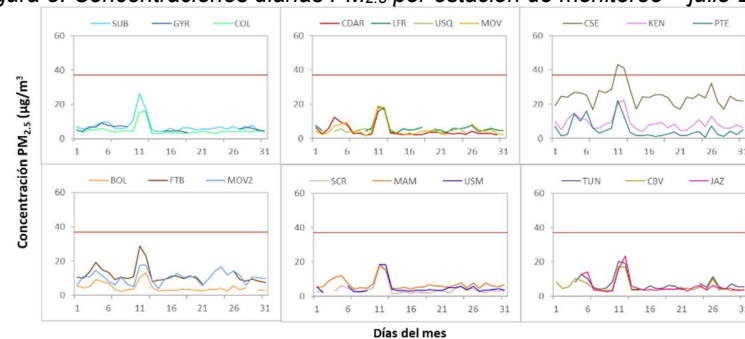
Figura 5. Concentraciones diarias PM 2.5 por estación de monitoreo – julio 2024.
