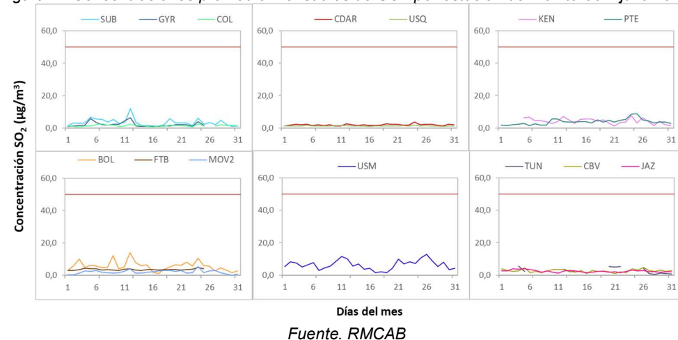
Figura 14. Concentraciones promedio mensuales de SO 2 por estación de monitoreo – julio 2024.
