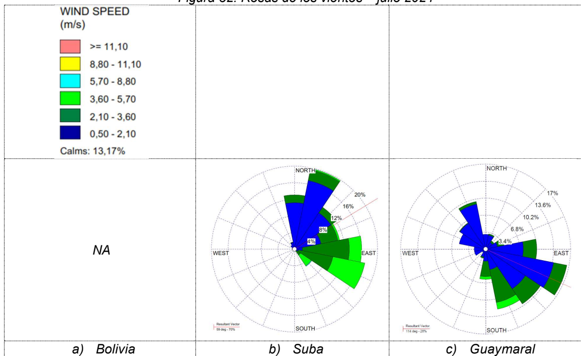
Figura 32. Rosas de los vientos – julio 2024
