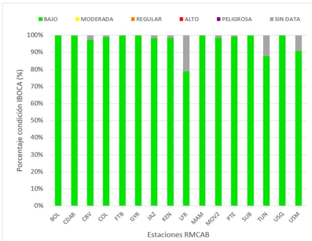
Figura 24. IBOCA para O3 por estación – julio 2024
