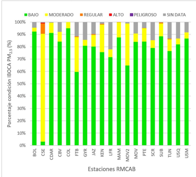
Figura 23. IBOCA para PM2.5 por estación – julio 2024
