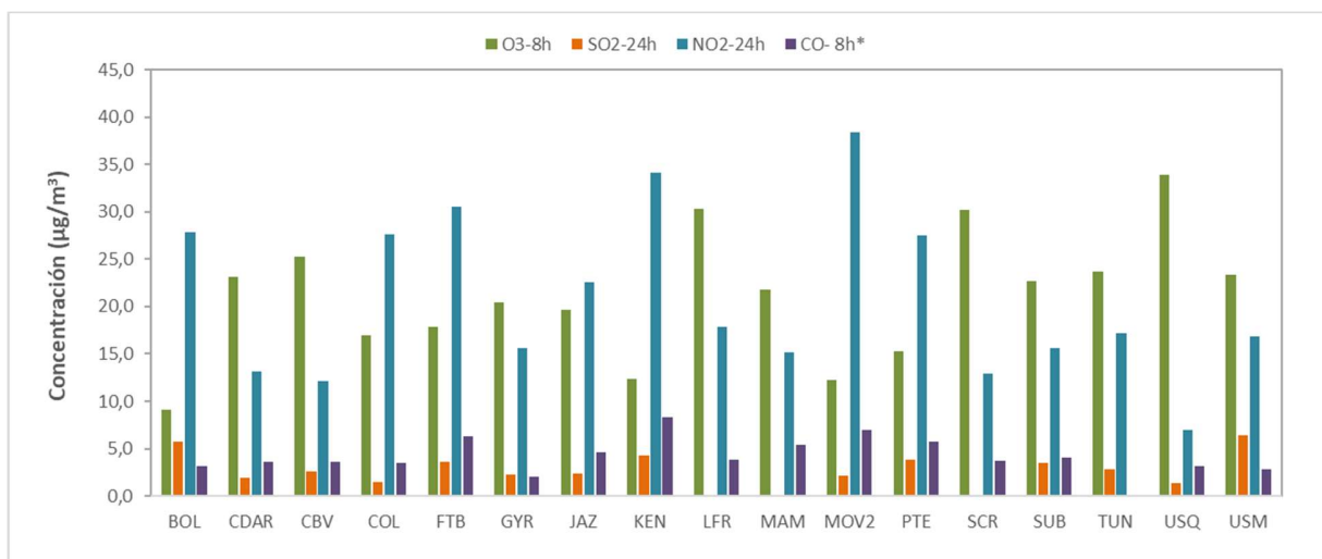
Figura 9. Concentraciones mensuales de gases (O 3 , SO 2 , NO 2 y CO) por estación de monitoreo – julio 2024.
