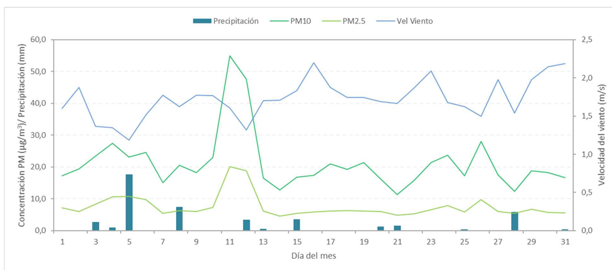
Figura 6. Promedio de concentración PM_{10} y PM_{2.5} , precipitación y velocidad del viento a nivel ciudad – julio 2024
