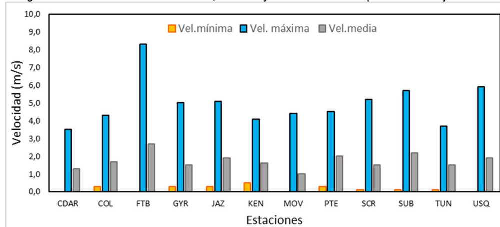
Figura 31. Velocidad del viento media, máxima y mínima absolutas por estación – julio 2024.
