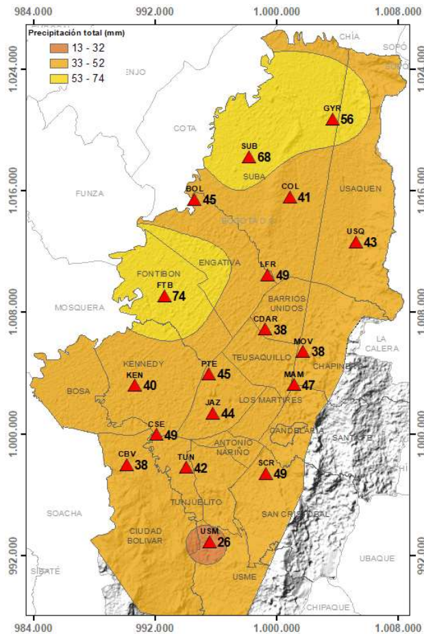
Figura 26. Mapa de la precipitación mensual total (mm) – julio 2024
