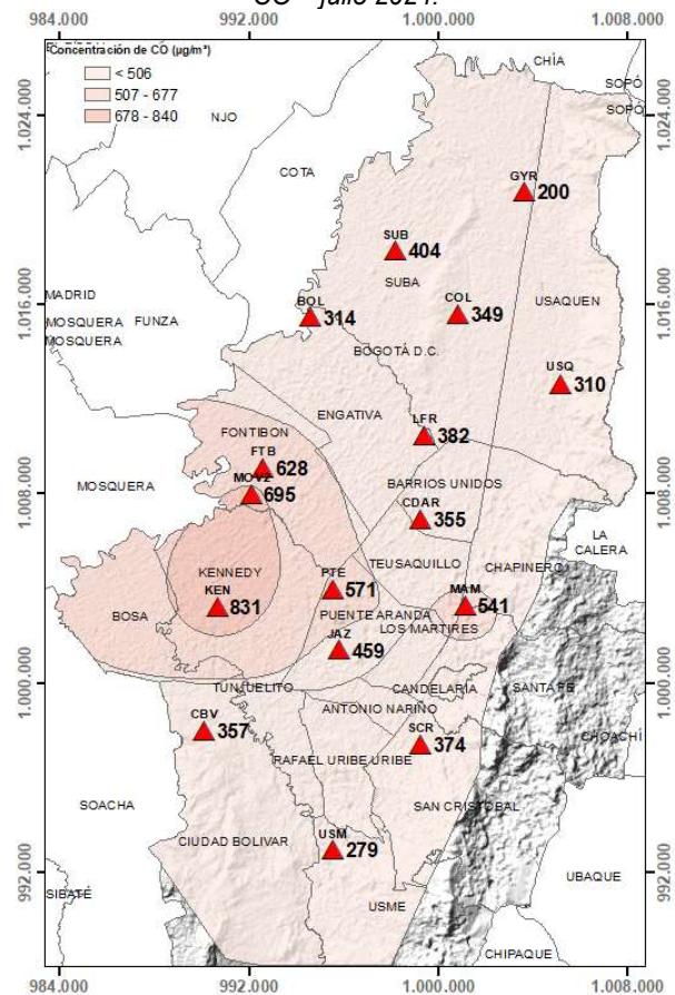
Figura 17. Distribución espacial concentraciones mensuales CO – julio 2024.
