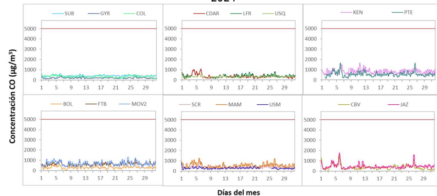
Figura 18. Concentraciones media móvil 8 horas de CO por estación de monitoreo - julio 2024
