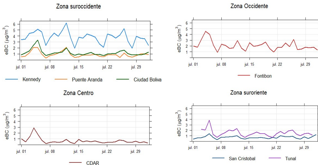
Figura 19. Comportamiento de las concentraciones diarias de eBC para julio de 2024
